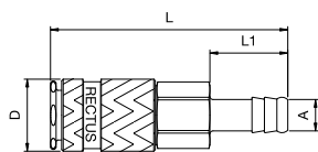
Schlauchanschluss
