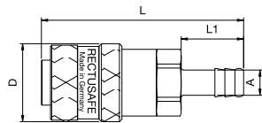
Schlauchanschluss
