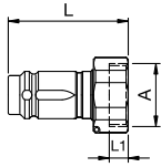
Innengewinde
